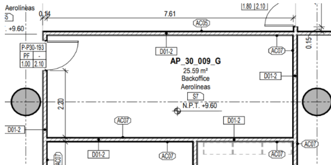
PLANTA P30
