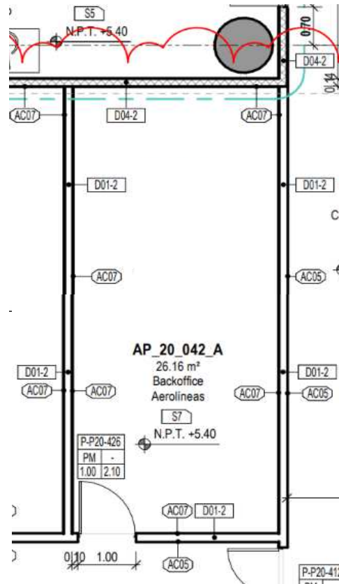
PLANTA P20
